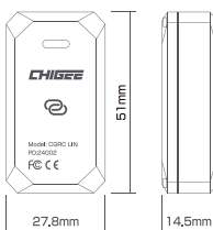
■ CGRC LINモジュール寸法
